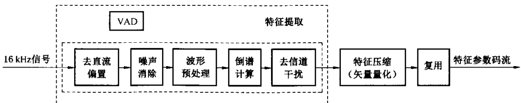
图 29 识别特征参数编码框图
