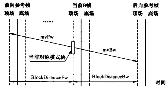
b) field_pic_flag 等于 1 时的对称模式
