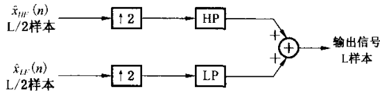
图 65 低频和高频信号合成
