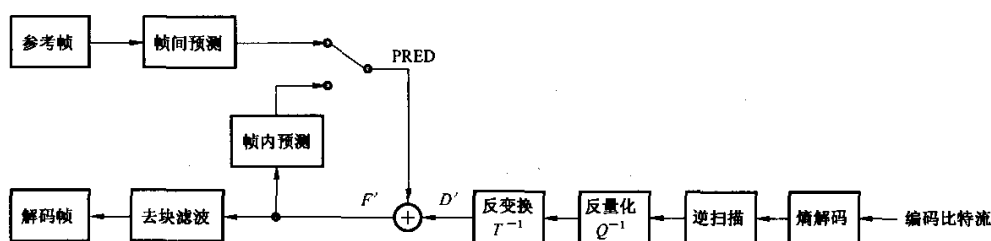
图 13 解码流程示例
