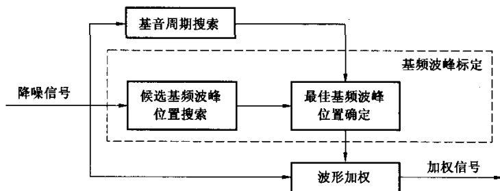
图 52 波形预处理原理框图
