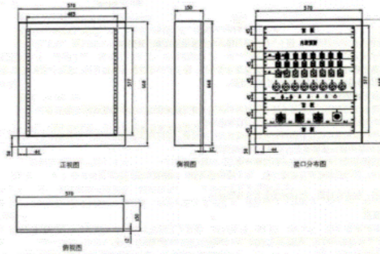
图3 舞台接口箱基本尺寸
