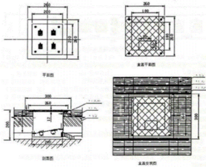
图5 舞台地板接线盒安装示意图
