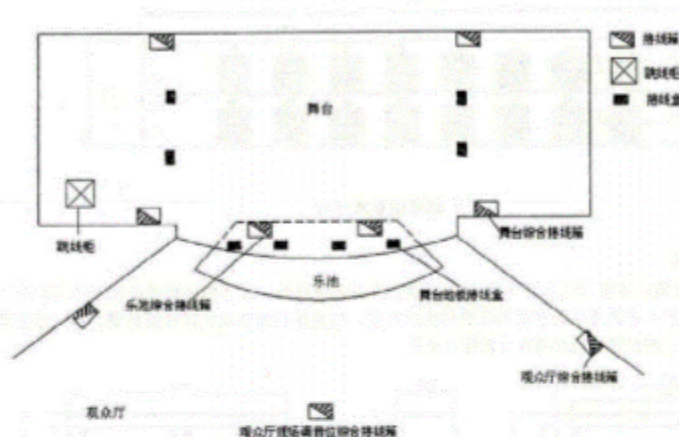
图1 舞台接口箱、地板接线盒位置示意图
