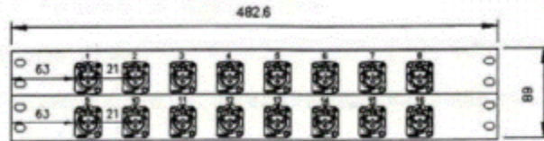
图2 跳线板基本尺寸
