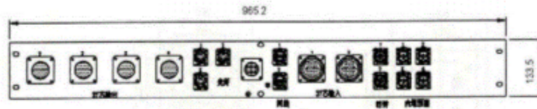
图4 观众厅接口箱基本尺寸
